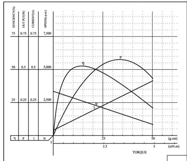
MODEL: DSD-280RA-2865
