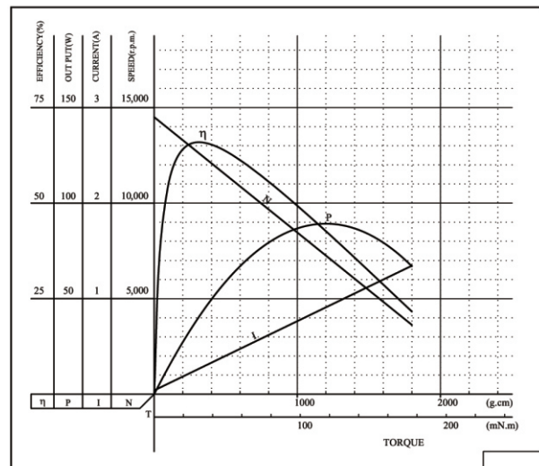
MODEL: DSD-5512SP-09210
