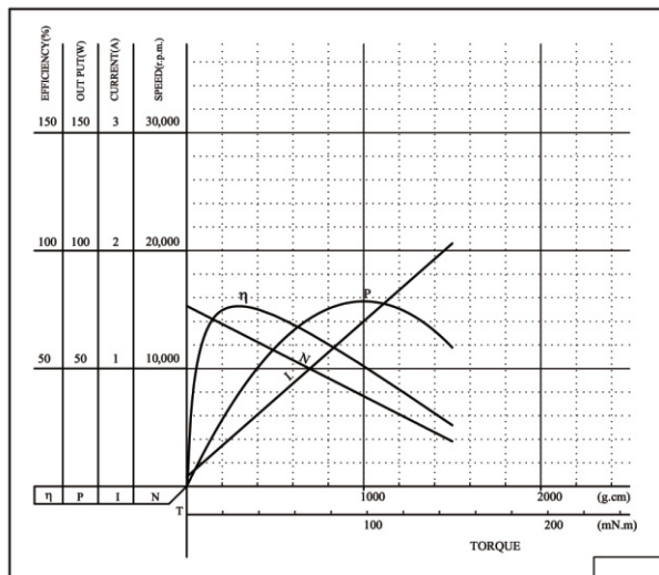
MODEL: DSD-5512SP-1595
